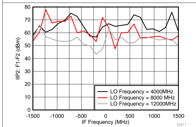
图 11. IIP2: F1-F2 Across LO Frequency for Internal LO Mode
