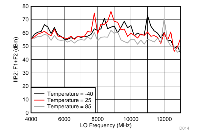
图 16. IIP2: F1+F2 Across LO Frequency for External LO Mode
