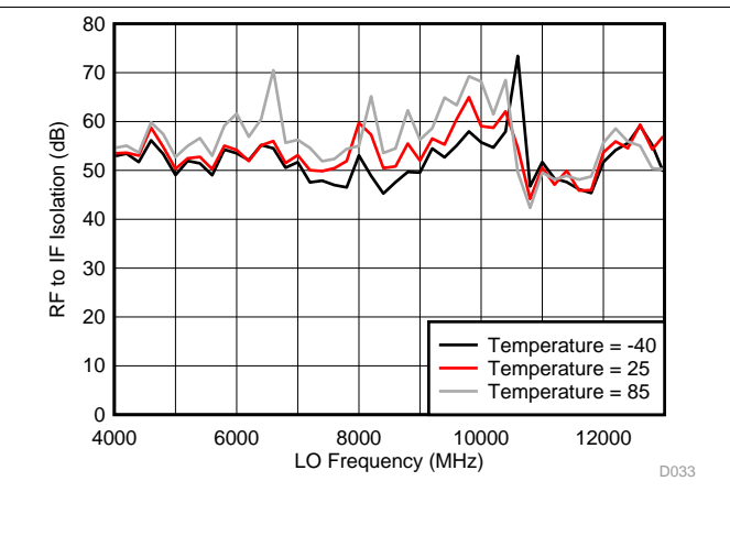
图 36. RF to IF Isolation
