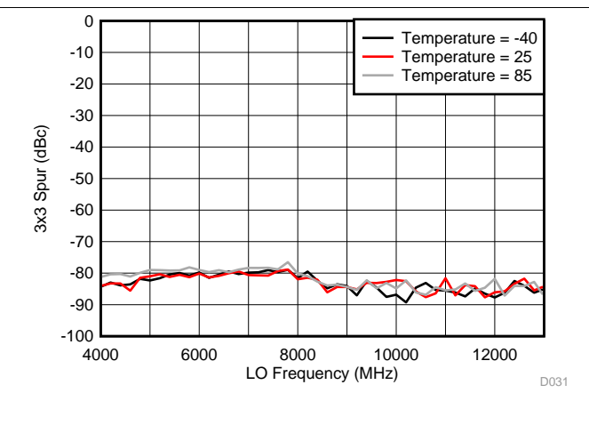
图 34. 3x3 Spur for Internal LO Mode
