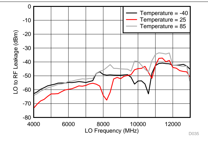
图 38. LO to RF Leakage Level: Internal LO Mode
