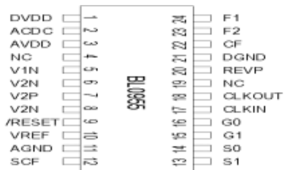
SSOP24
